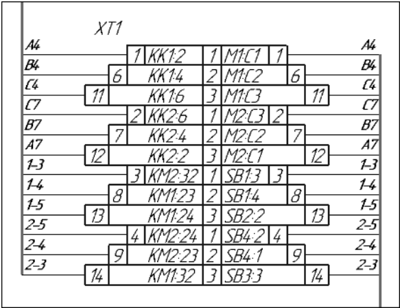
Рис. 22.19. Многоярусный клеммник на схеме Э4
