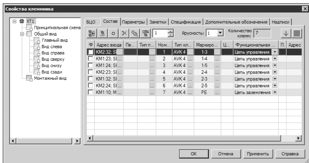
Рис. 26.10. Состав клеммника
