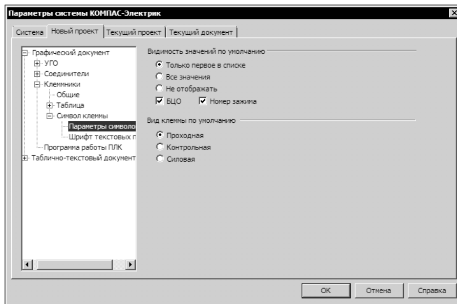
Рис. 19.7. Настройка параметров символов клемм
