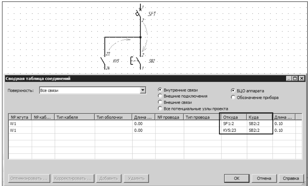
Рис. 26.9. Соединение между зажимами трех аппаратов
