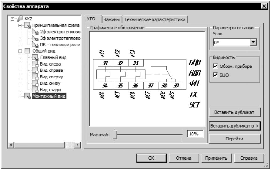
Рис. 21.12. Диалог Свойства аппарата на уровне Монатжный вид
