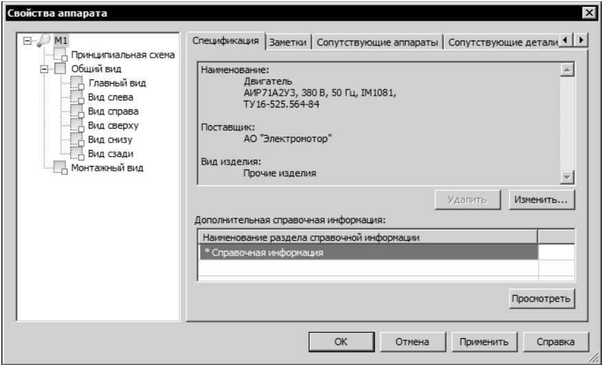
Рис. 21.6. Диалог общих свойств аппарата
