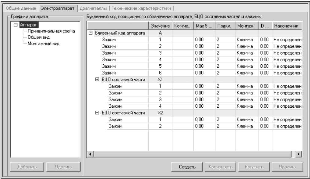
Рис. 6.6. Уровень Аппарат во вкладке Электроаппарат
