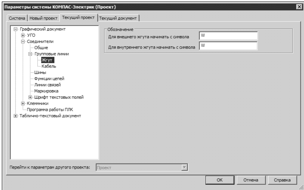
Рис. 26.4. Настройка соединителей. Обозначения жгутов.
