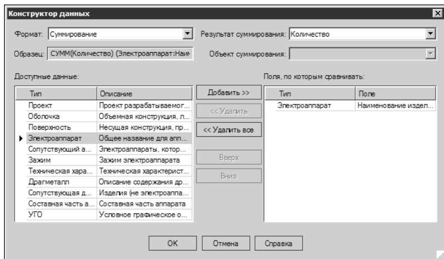
Рис. 14.20. Данные, отображаемые в столбце Количество .
