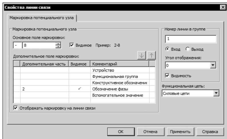
Рис. 22.7. Диалог свойств линии связи
