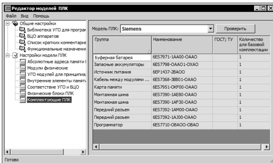
Рис. 7.14. Комплектующие ПЛК
