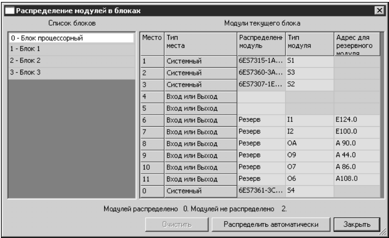
Рис. 24.4. Распределение модулей в блоках
