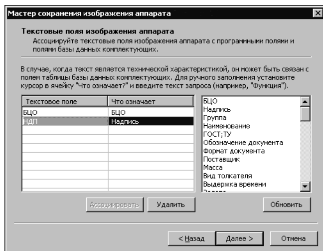
Рис. 11.20. Ассоциация текстовых полей
