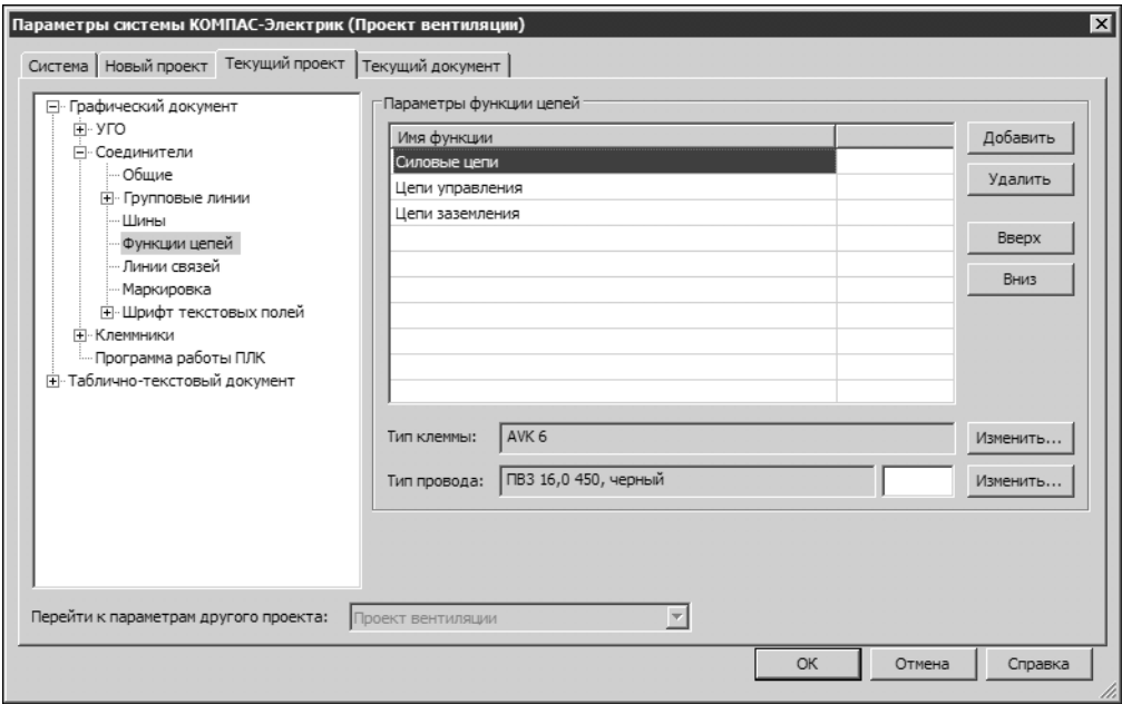
Рис. 19.2. Настройка функций цепей
