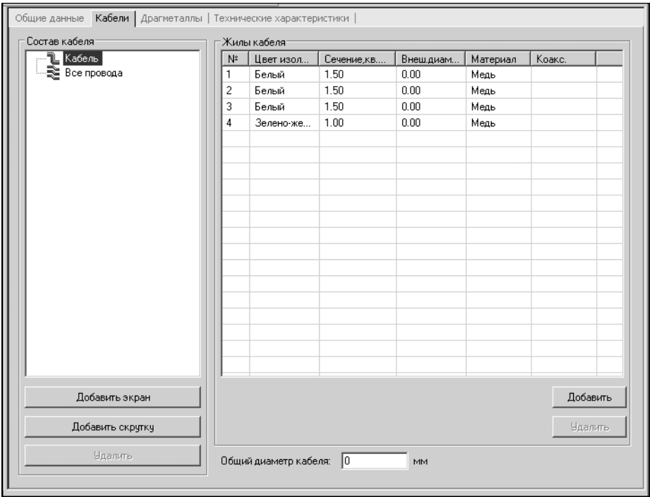
Рис. 6.14. Вкладка Кабели
